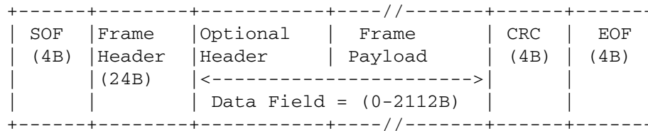
Fig. 16 FC Frame Format
